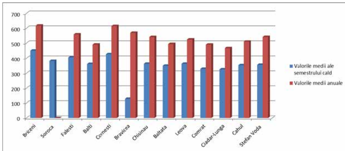
Fig. 3.2. Repartiția teritorială a valorilor medii de precipitații (mm) din semestrul cald și anuale
