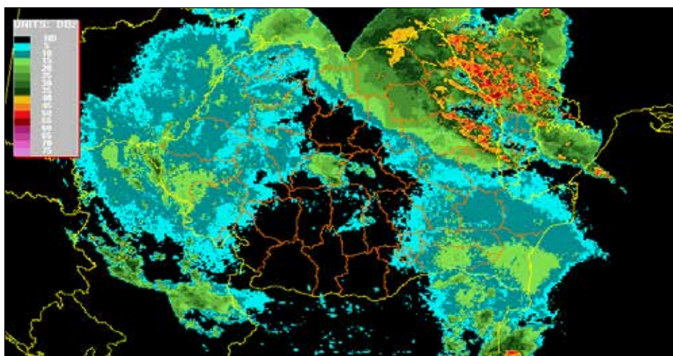
Fig. 3.27. Harta complexă-radar (reflectivitate maximă în decibeli) la momentul intensității maxime a ploilor torențiale pe 18.08.2005 ora 20.07 UTG.
