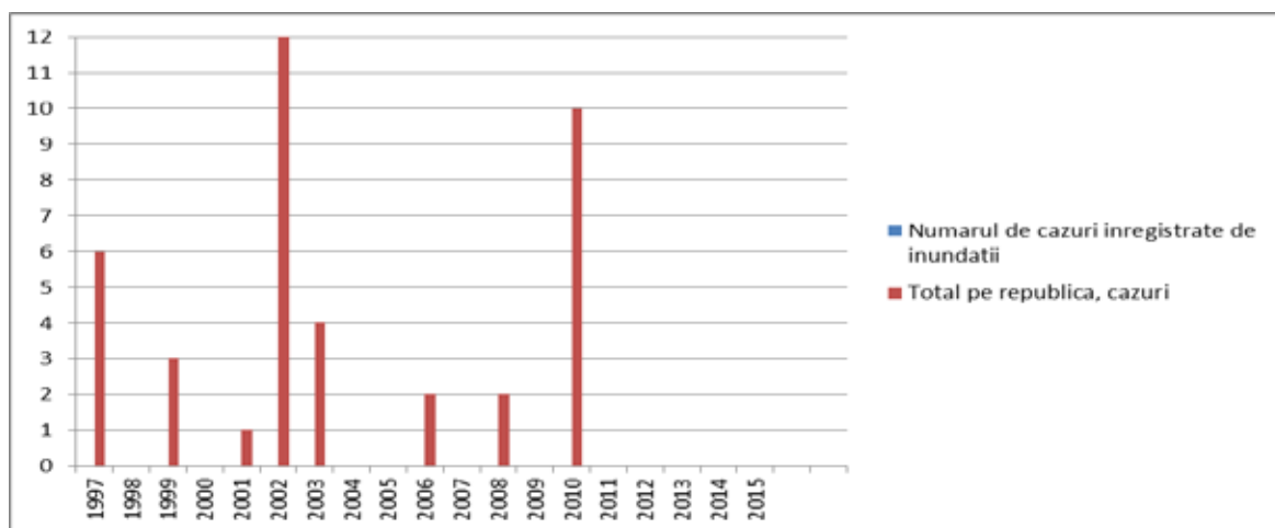
Fig. 3.28. Frecvența anuală a inundațiilor declanșate de ploile torențiale în semestrul cald al anului cu prejudicii semnificative înregistrate (1997-2015)
