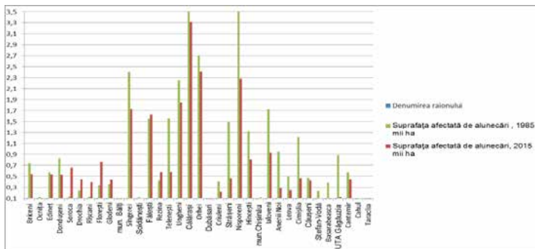
Fig. 3.32. Suprafața afectată de alunecări de teren în profil administrativ-teritorial (1985 și 2015)
