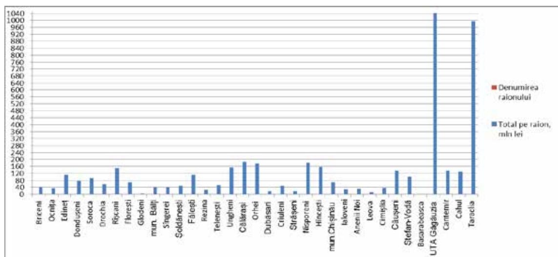
Fig. 3.18. Variația prejudiciilor cauzate de ploile torențiale în semestrul cald al anului în profil administrativ-teritorial (1997-2015)
