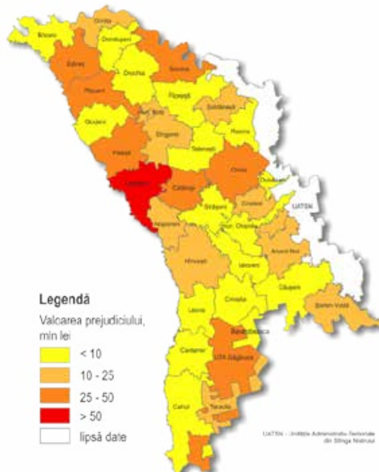
Fig. 3.20. Prejudiciile cauzate de ploile torențiale (1997-2015). Mai
