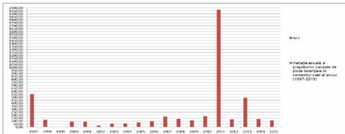
Fig. 3.16. Variația anuală a prejudiciilor cauzate de ploile torențiale în semestrul cald al anului (1997-2015)
