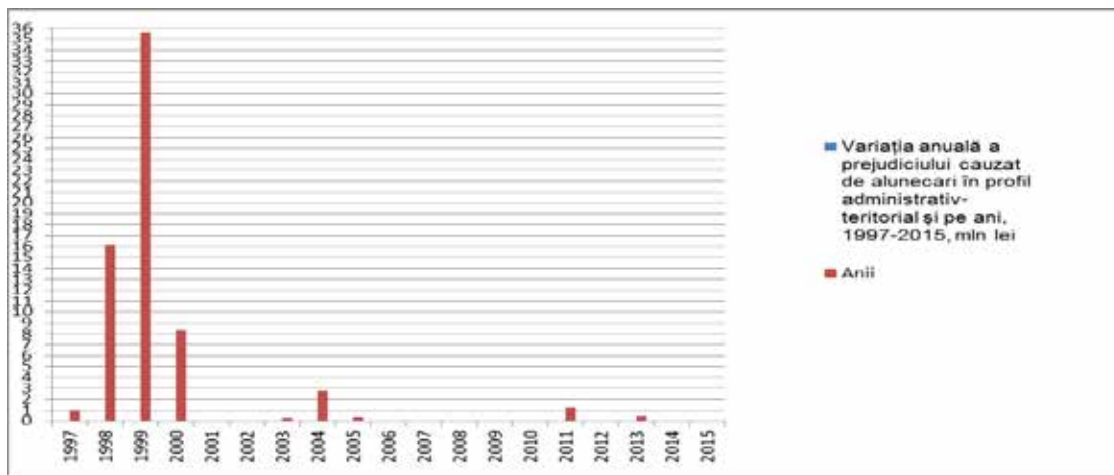
Fig. 3.35. Variația anuală a prejudiciilor semnificative cauzate de alunecări de teren
