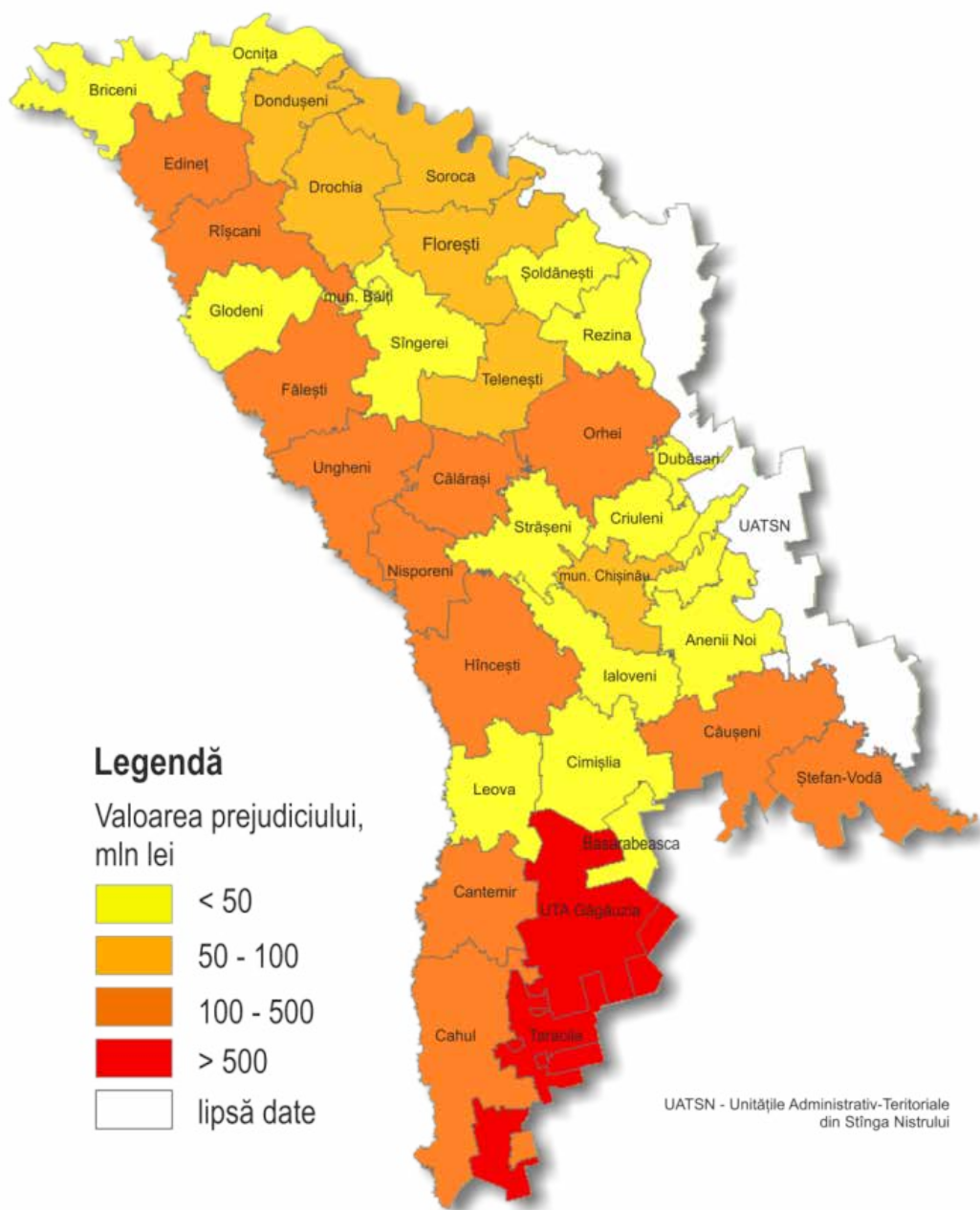
Fig. 3.25. Expunere a teritoriului RM față de riscul ploilor torențiale din semestrul cald al anului (1997-2015)
