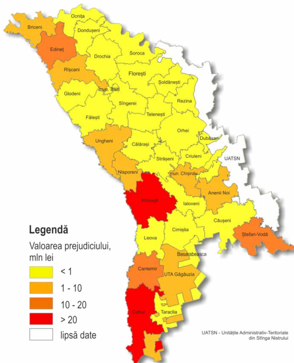
Fig. 3.31. Expunerea teritoriului republicii în profil administrativ-teritorial față de riscul inundațiilor declanșate de ploile torențiale în semestrul cald al anului (1997-2015)
