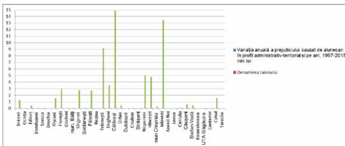
Fig. 3.37. Prejudiciul semnificativ înregistrat în profil administrativ-teritorial (1997-2015)
