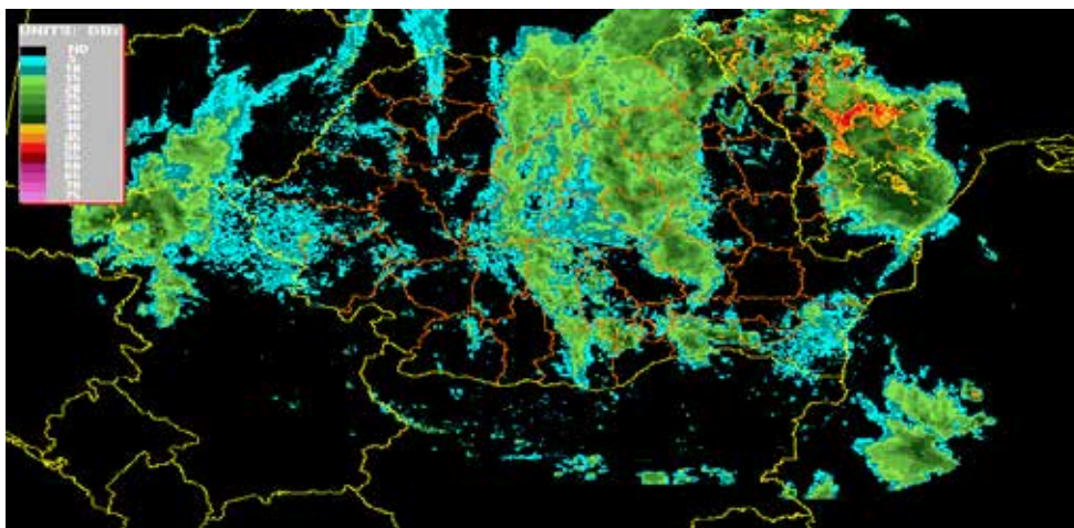
Fig. 3.26. Harta complexă-radar (reflectivitate maximă în decibeli) la momentul intensității maxime a ploilor torențiale pe 7.08.2005 ora 11.27 UTG.
