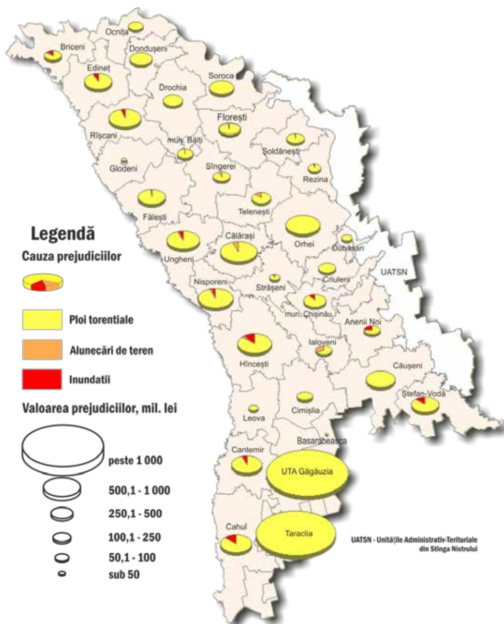
Fig. 3.39. Harta complexă a prejudiciul total al riscurilor studiate și cota-parte a prejudiciilor cauzate de fiecare risc în profil administrativ-teritorial (1997-2015)
